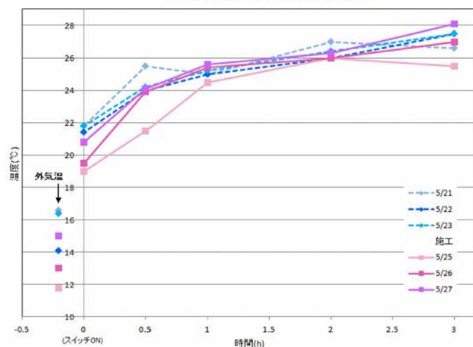
■工事前後の床表面温度比較■
